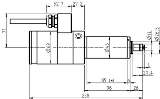
寸法図
